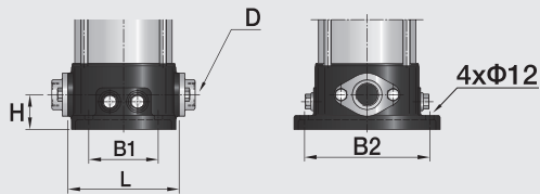
Круглый фланец (F)
