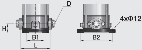
Овальный фланец (N)
